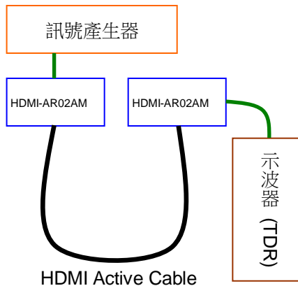
圖 1: HDMI Active cable 測試示意圖
