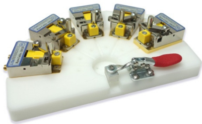
圖一: LT-100R-20GD-5P 5 對裸線夾具
