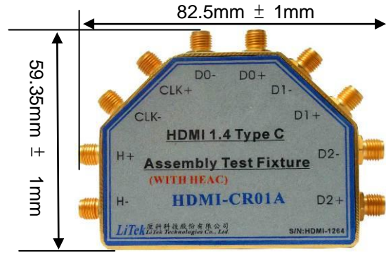
Fig 3: HDMI-CR01A 尺寸圖。
