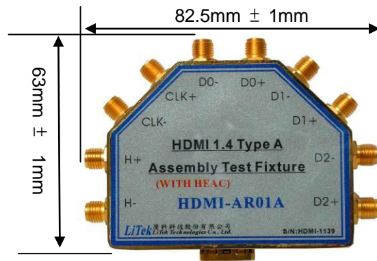
圖 3: HDMI-AR01A 尺寸圖
